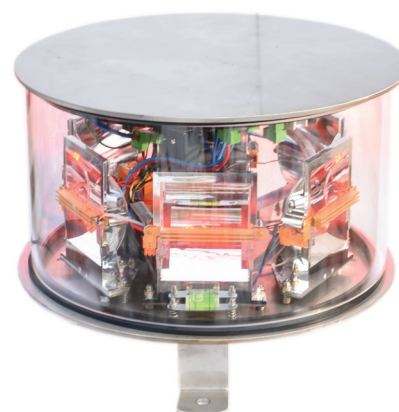
Mittlere Intensitäts-Hindernislampe MSL-2010
